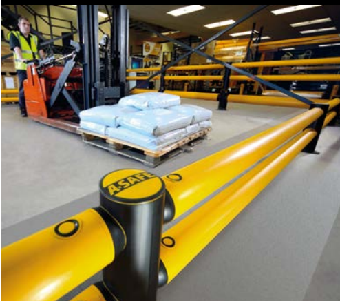
mFlex Rail Vloerniveau
